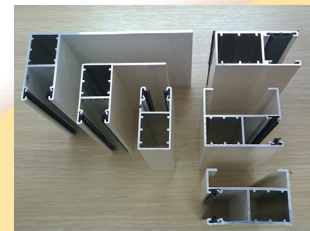
Verschillende type zijgeleiders
